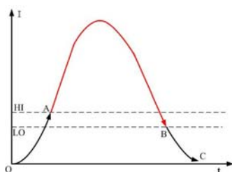
图 2: 电流继电器 2 工作原理
