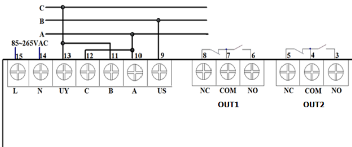
三相三线制接线
