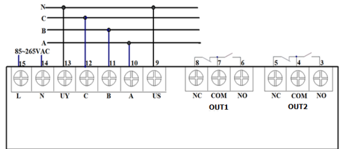
三相四线制接线
