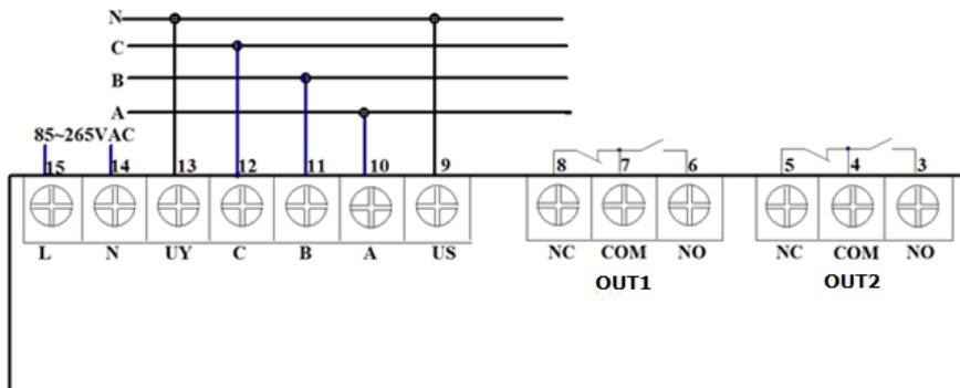
三相四线制接线
