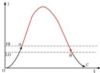
图 2: 电流继电器 2 工作原理
