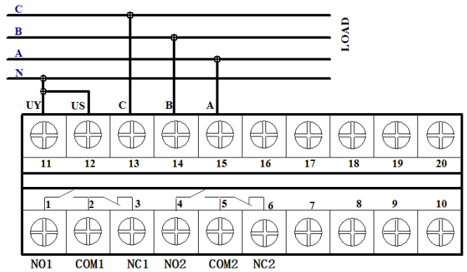
三相四线制接线
