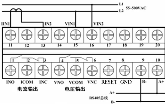
端子接线图
