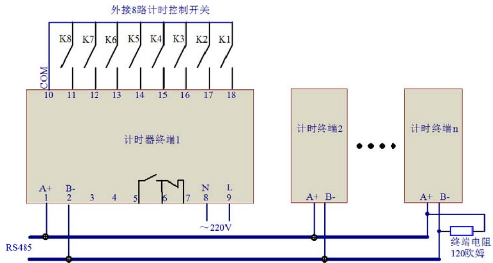
图1：端子接线图
