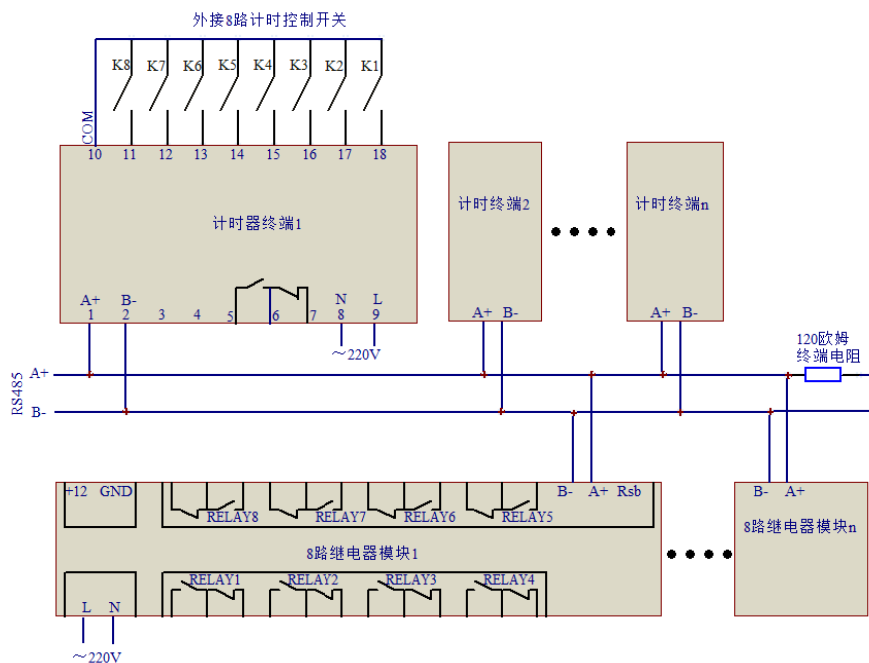
图 2：配合 8 路继电器模块接线
